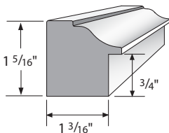
Backband VER281
