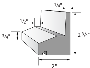
Water Table VERWT01 ■ 18'
